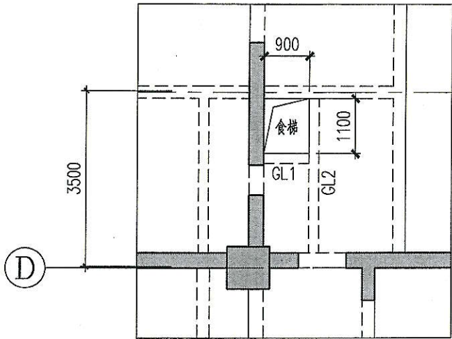
增加电梯处局部平面图
